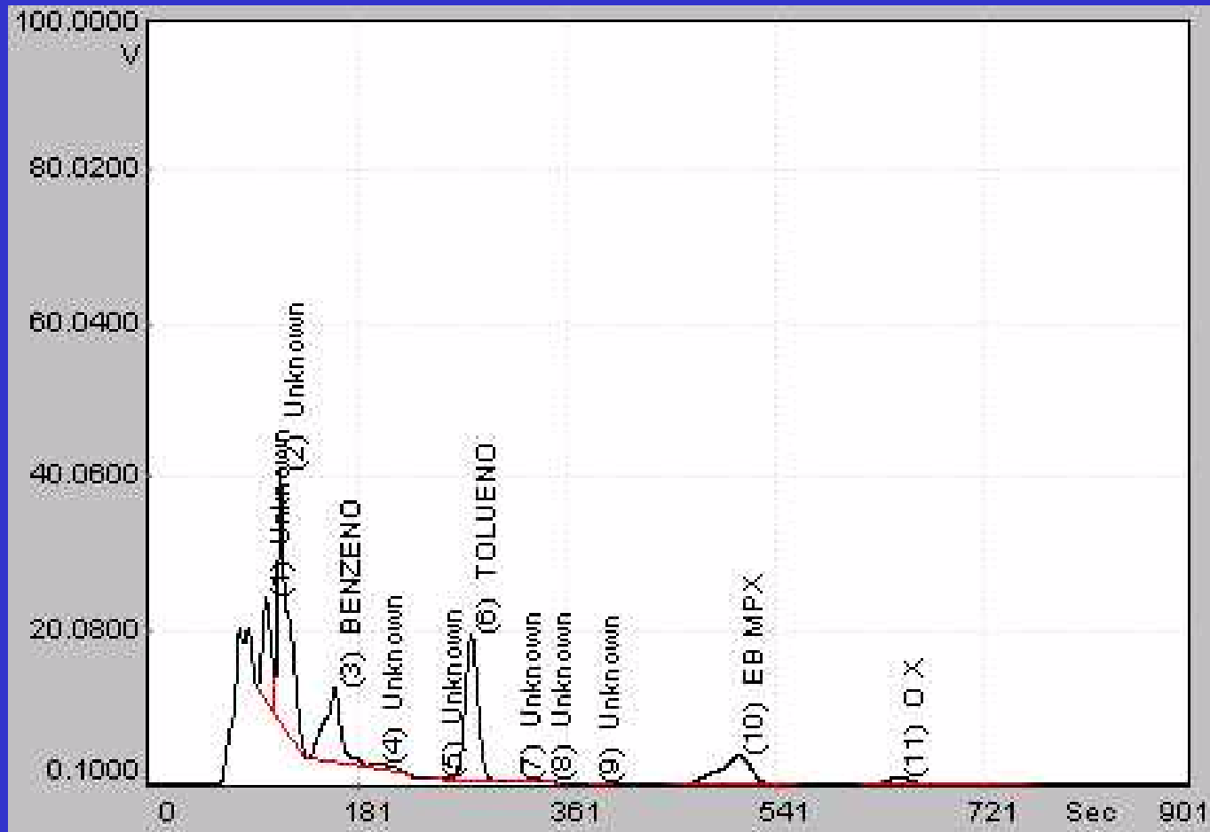
Cromatógrafo: Perkin- Elmer Voyager
