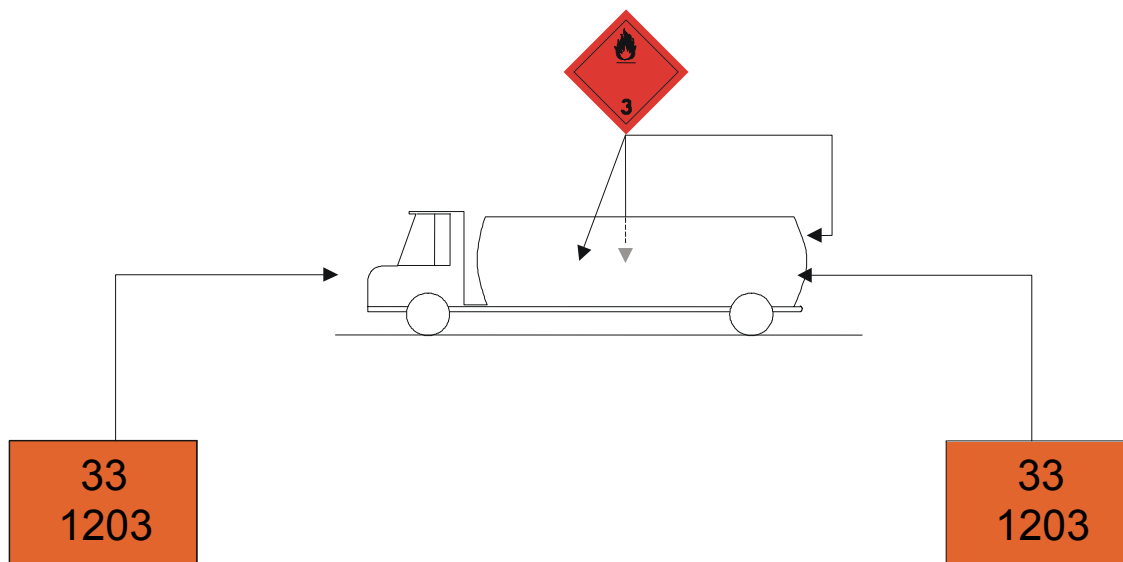
Fig. 2 Veículo-tanque carregado com dois produtos perigosos da mesma classe ou subclasse (*):
